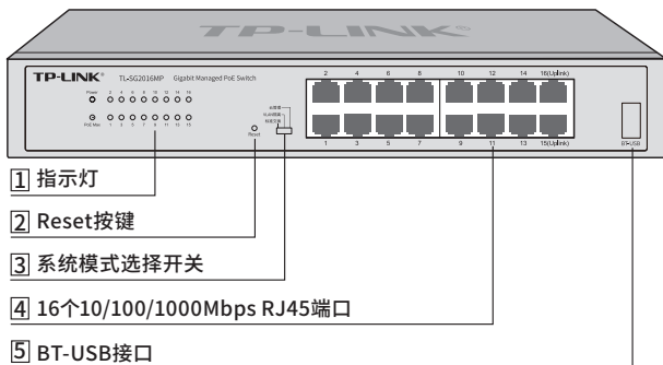
图1-2 TL-SG2016MP前面板示意图
