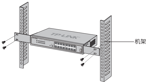
图2-3 机架安装示意图
