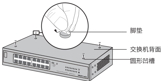
图2-1 桌面安装示意图
